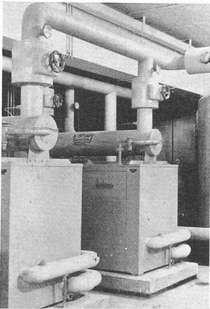
Fig. 4. — Centrale frigorifique, avec deux générateurs d'eau glacée Chrysler.
