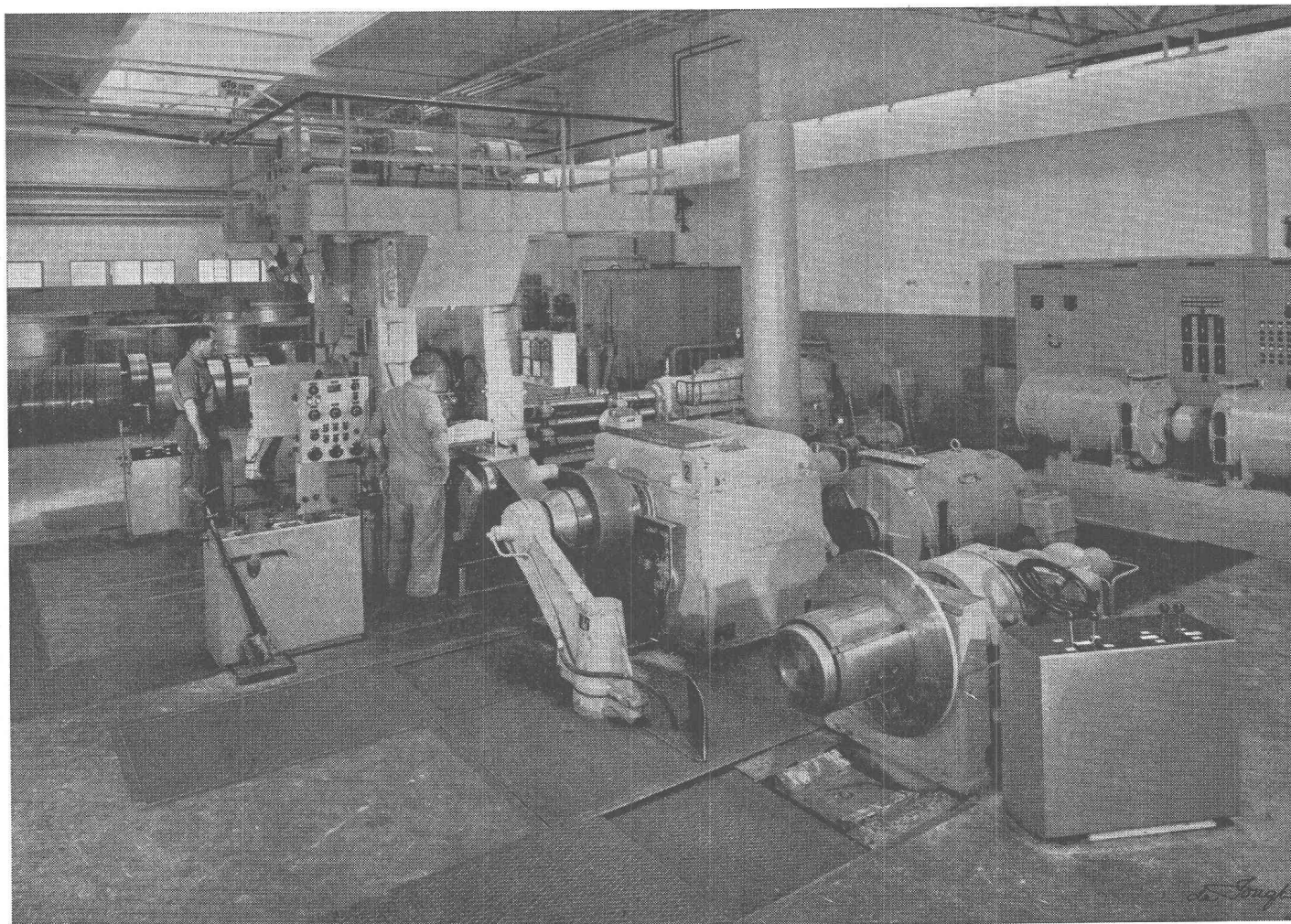
Laminioir quarto réversible à commande électronique pour le laminage de feuillets de fer. (Photo prise au Département de laminage de la S.A. des Câbleries et Tréfileries de Cossonay)
