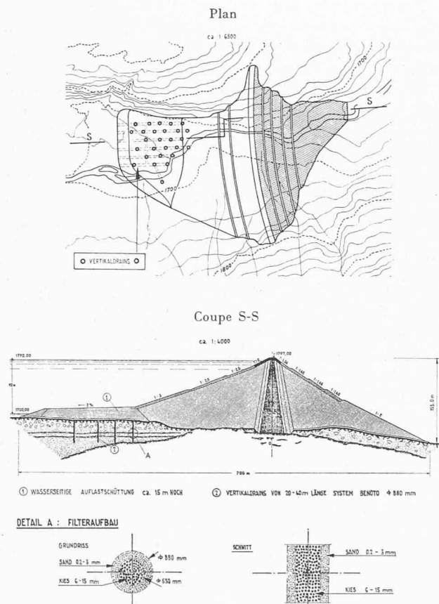
Fig. 16. — Drains de sable digue Göscheneralp.
