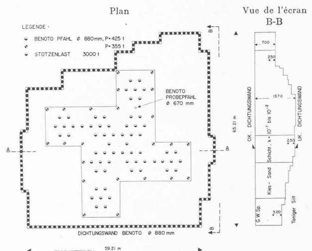
Fig. 14a. — Ecran étanche, chantier « Palme », à Zurich.
