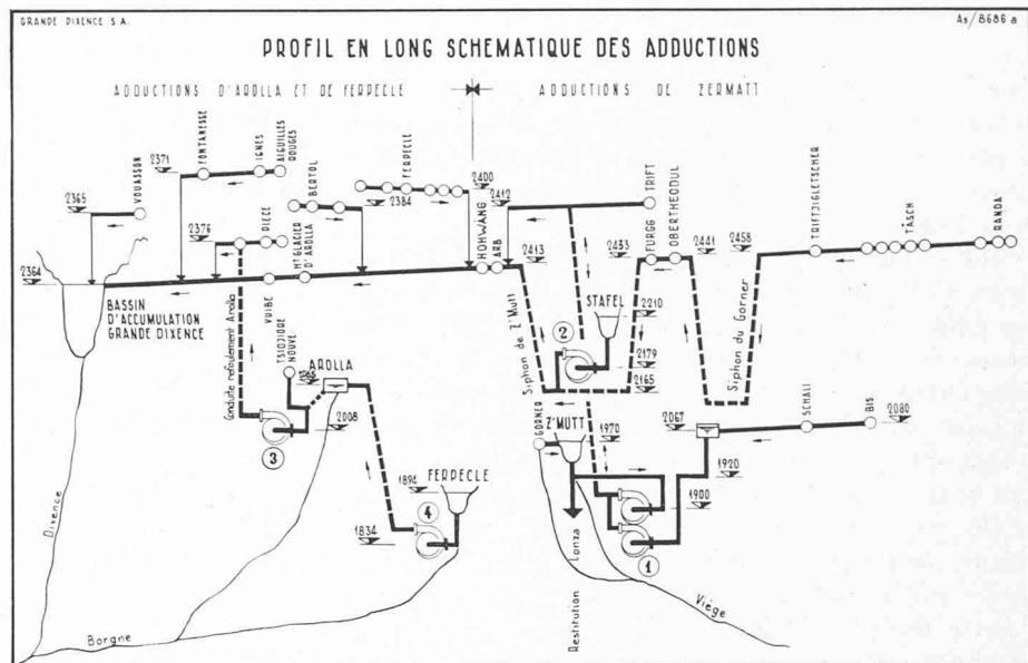
Fig. 2. — Les galeries d'aménée latérales débouchant dans le collecteur sont représentées au-dessus de celui-ci pour la clarté du schéma.
