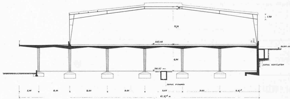
Fig. 8. — Projet exécuté, coupe transversale sur un pavillon.
