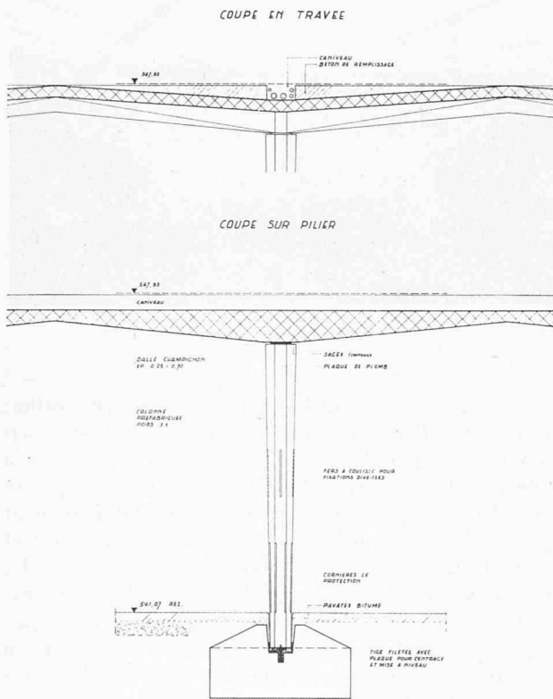
Fig. 9. — Détail d'un pilier et de la dalle-champignon.
