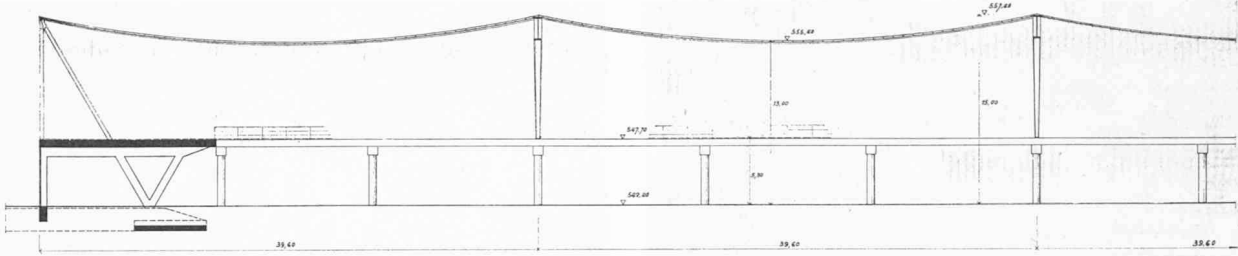
Fig. 4. — Toiture suspendue, coupe longitudinale.
