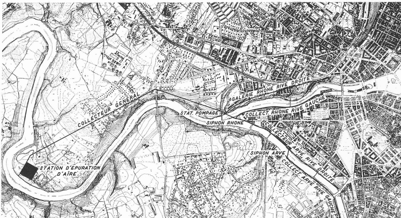
Fig. 1. — Plan d'ensemble.
