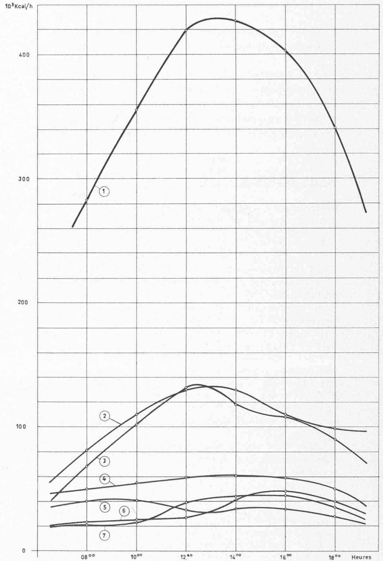
Fig. 5. — Graphique des puissances frigorifiques.
