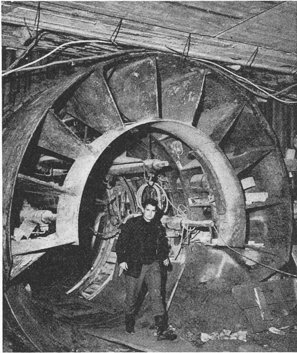
Fig. 7. — Le bouclier, à son arrivée dans le tunnel transversal.
