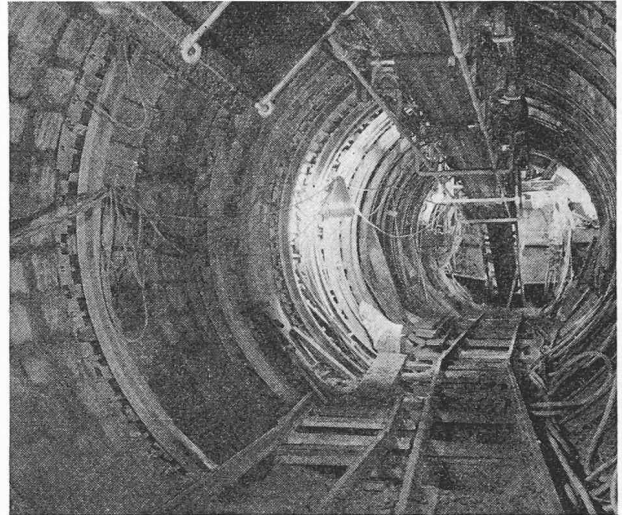
Fig. 8. — Vue du revêtement immédiatement derrière le bouclier.
