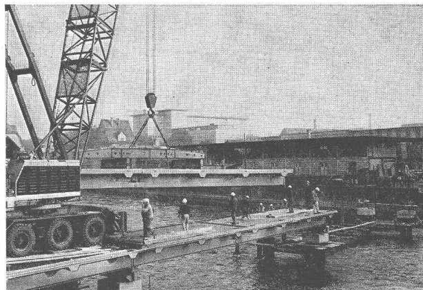
Pont système « Rheinstahl » sur la Limmat à Zurich. Longueur 81 m, 2 voies. Durée du montage : 15 heures.
