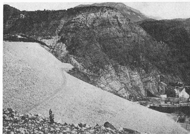
Fig. 44. — Digue de Serre-Ponçon. Vue du parement aval.
