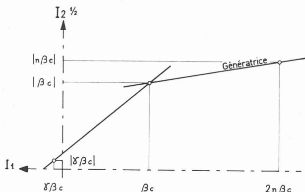
Fig. 18. — Génératrice de la surface tronconique de rupture.
