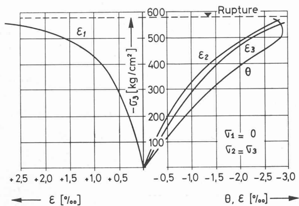
Fig. 8. — Déformations d'une éprouvette soumise à une charge biaxiale croissante ( \sigma_1 = 0, \sigma_2 = \sigma_3 ) [9].
