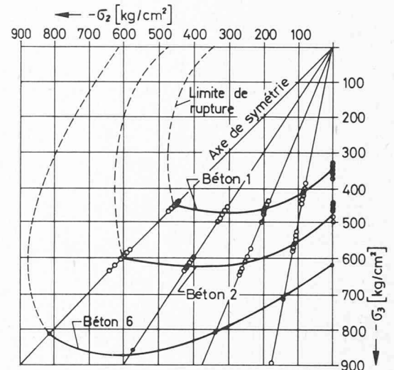
Fig. 13. — Essais de rupture en compression biaxiale [9].
