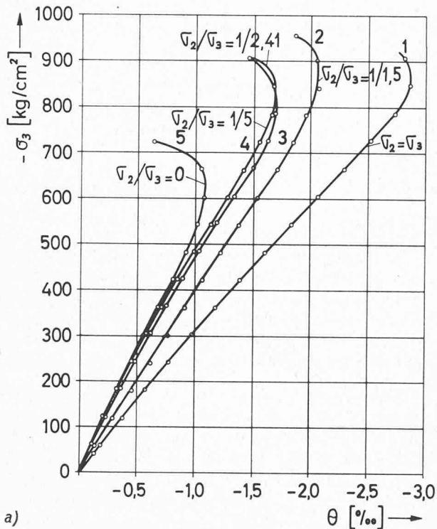
Fig. 21. — Variations de volume ( \theta ) lors d'essais biaxiaux sous charge croissante pour plusieurs rapports de \sqrt{\sigma_2}/\sigma_3 . a) \theta exprimé en fonction de \sigma_3 [9]; b) \theta exprimé en fonction de \bar{\sigma} .
