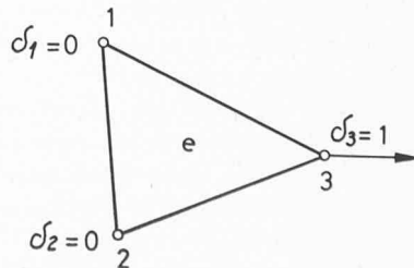
Fig. 25. — Élément dont un nœud est soumis à un déplacement unitaire.
