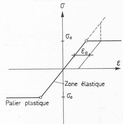
Fig. 28. — Schéma « contrainte-déformation » des armatures.
