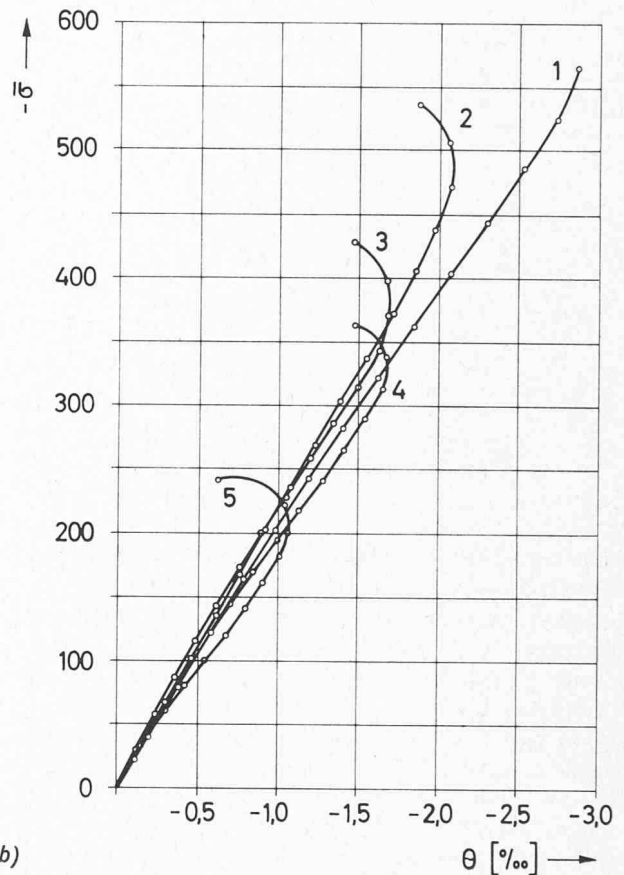
Fig. 21. — Variations de volume ( \theta ) lors d'essais biaxiaux sous charge croissante pour plusieurs rapports de \sqrt{\sigma_2}/\sigma_3 . a) \theta exprimé en fonction de \sigma_3 [9]; b) \theta exprimé en fonction de \bar{\sigma} .
