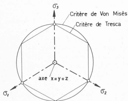
Fig. 5. — Sections droites des critères de von Misès et de Tresca.
