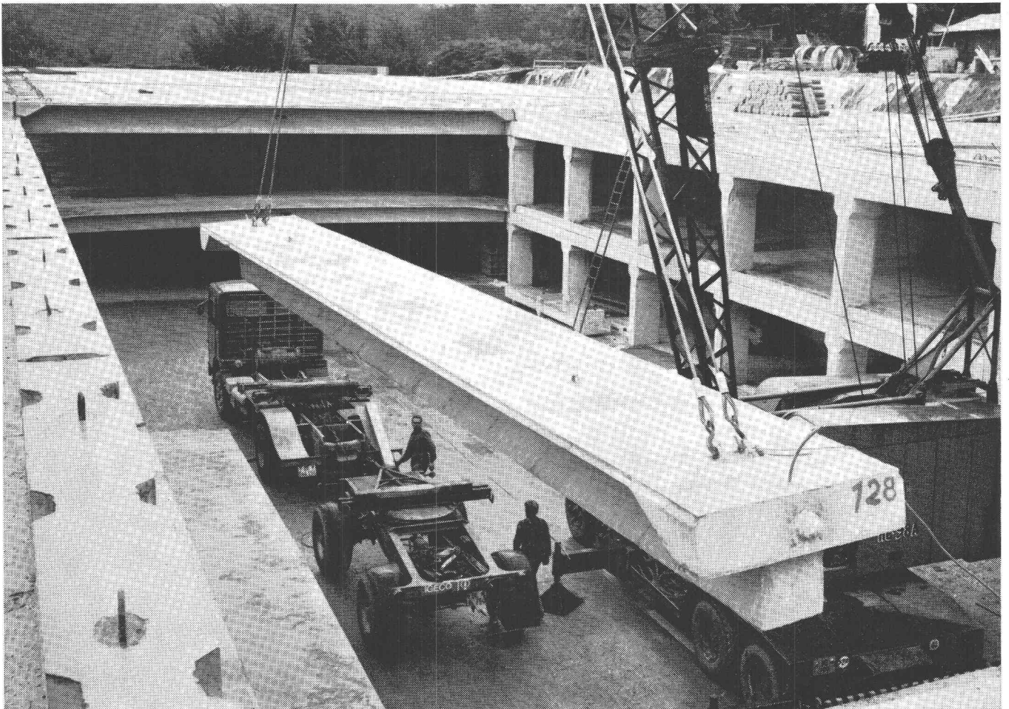
Parking souterrain des Grand'Places, Fribourg Fabrication et montage : IGECO S.A., Etoy Photo : Marc Liguori
