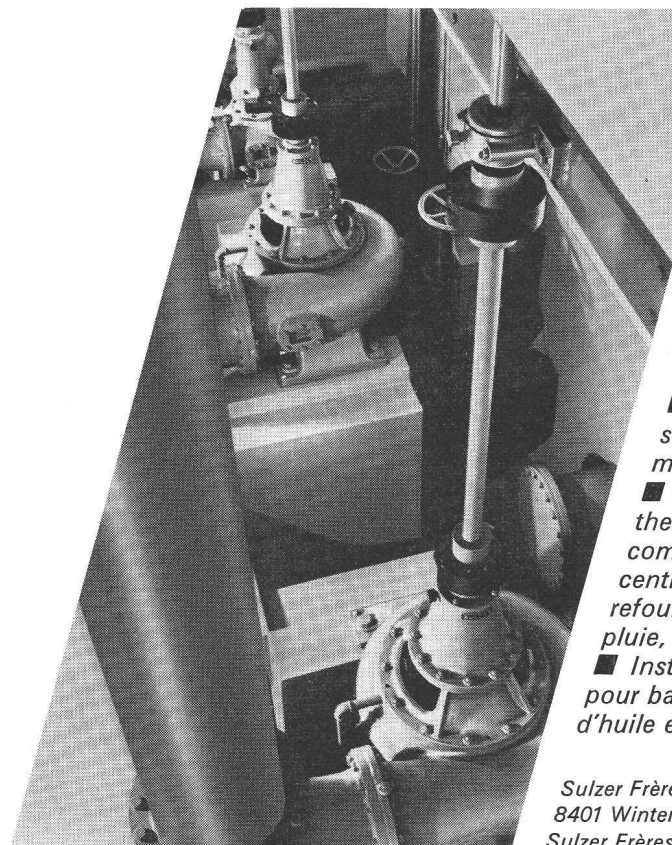
Pompes verticales, Sulzer à eaux usées dans la station d'épuration de Küssnacht/Erlenbach
