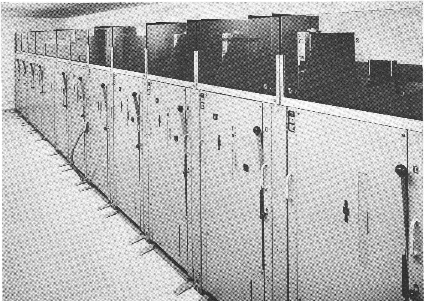
Installation haute tension à isolation compacte type PB 204, tension nominale 12 kV.
