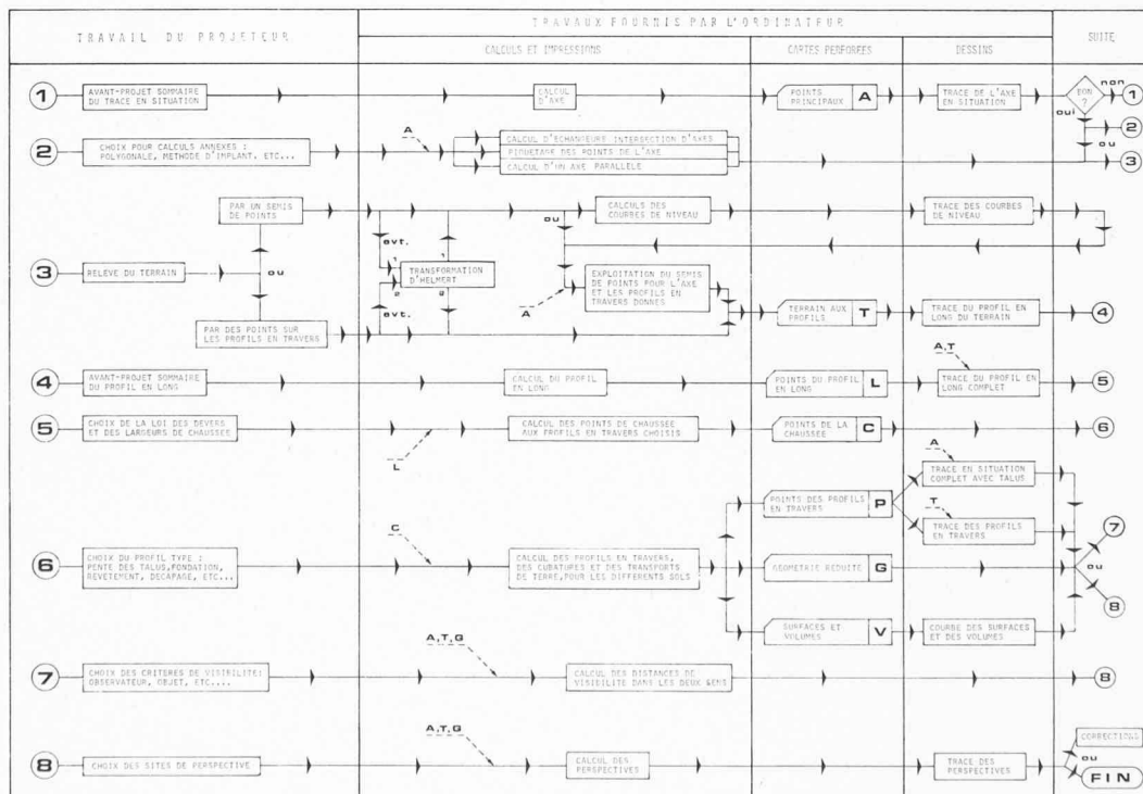
Fig. 1. — Schéma d'utilisation.
