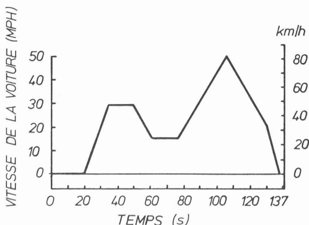
Fig. 22. — Cycle California (à répéter 7 fois).
