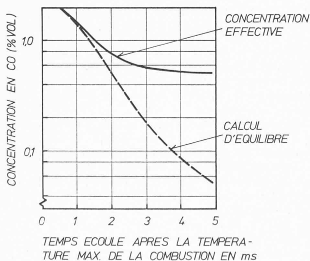
Fig. 9. — Evolution de la formation du CO lors de la combustion et de la détente.
