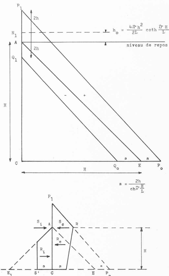
Fig. 1. — Diagramme de pression sur un obstacle vertical.
