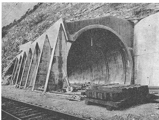
Fig. 101. — La pose des voies au portail de Seefels, du côté Bielle, en 1968. Au premier plan, l'ancienne simple voie à l'air libre encore en service.
