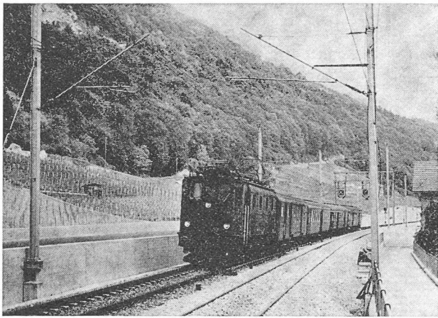
Fig. 96. — La double voie entre Douanne et Daucher au printemps 1975, peu avant sa mise en service. A gauche, la RN 5 et à droite, le nouveau chemin de rive (photo S. Jacobi).
