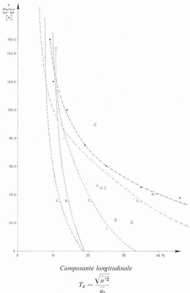
Profils relevés dans la nature A Davenport, mesures à Brookhaven B mesures à Sale Profils reproduits en soufflerie E soufflerie F+W, Emmen \varnothing 113 mm F soufflerie EPFZ \varnothing 80 mm G soufflerie EPFL-ISM \varnothing 16 mm H soufflerie EPFL-ISM \varnothing 10 mm
