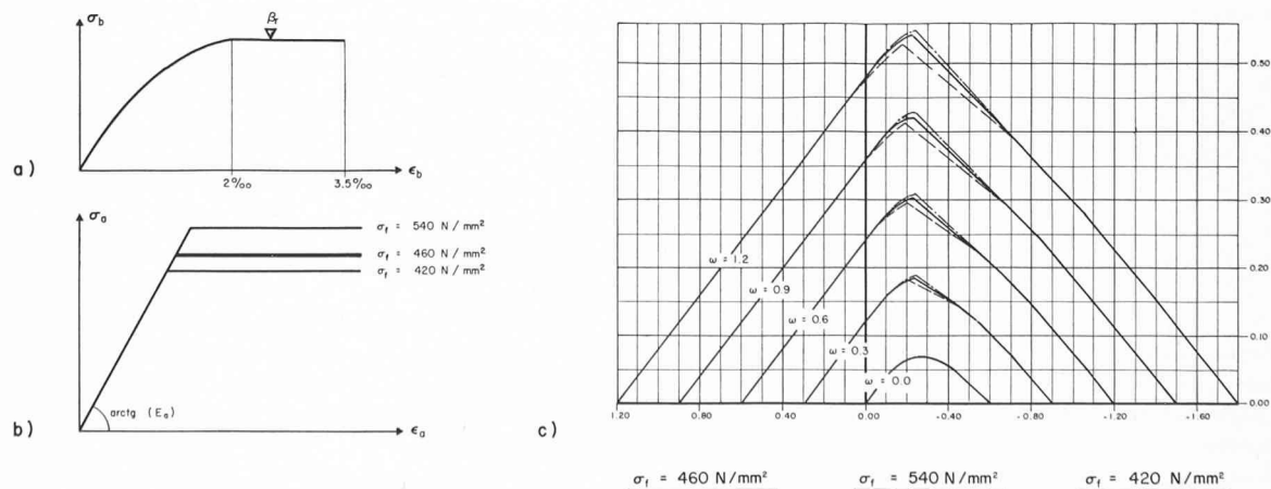
Fig. 12. — Lois \sigma - \epsilon selon DIN-CEB pour le béton a) et l'acier b); influence de la qualité de l'acier sur la résistance des sections c).
