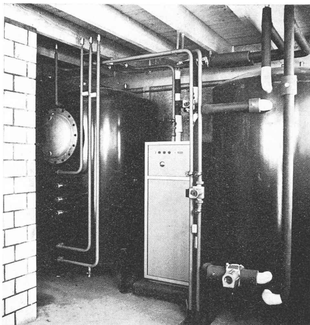
Chaufferie Promasol, alimentée par l'énergie solaire, avec pompe à chaleur et accumulateur permettant de bénéficier du tarif le plus avantageux.
