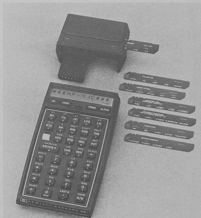
HP-41C et lecteur de cartes magnétiques. La calculatrice comporte quatre prises permettant d'enficher jusqu'à quatre modules (mémoire ou application), le lecteur de cartes, l'imprimante ou le lecteur de code optique.
