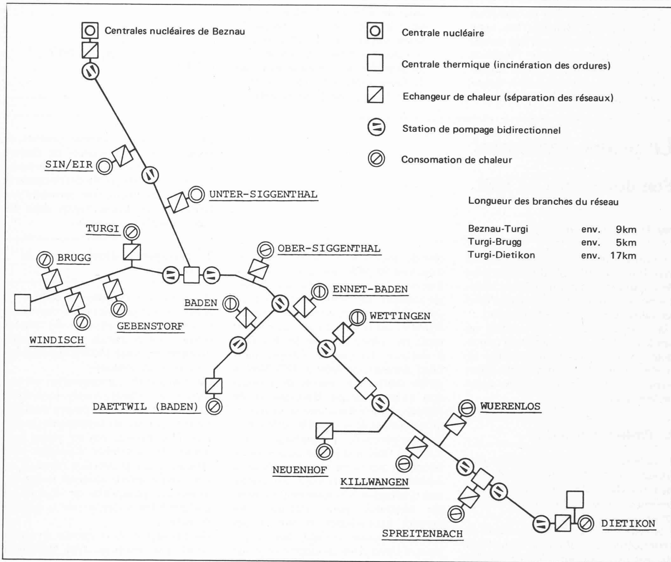
Fig. 2. — Transwaal. Production et distribution de chaleur.
