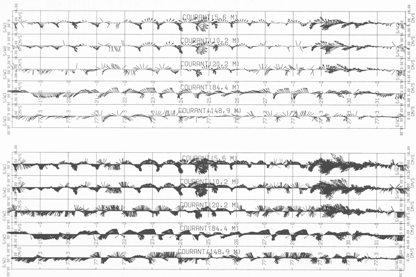
Fig. 7. — Diagramme vectoriel en bédons pour les mesures de courants à Saint-Sulpice du 18 au 31 mars 1977. a) Vecteurs observés chaque 10 minutes; b) Vecteurs moyennés sur 1 heure.
