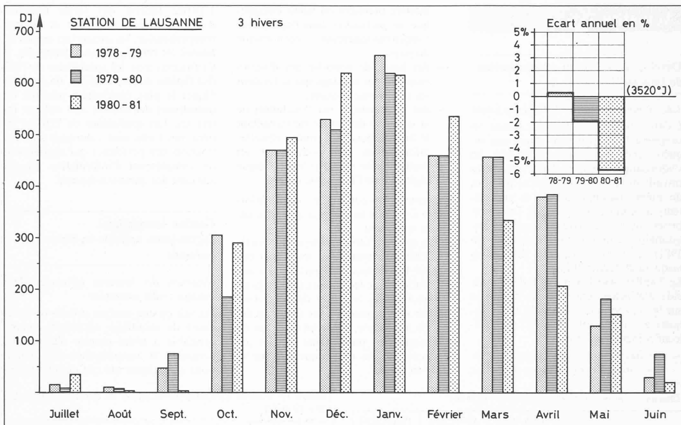
Fig. 2 — Degrés-jours mensuels et écarts annuels, calculés de juillet 1978 à juin 1981.
