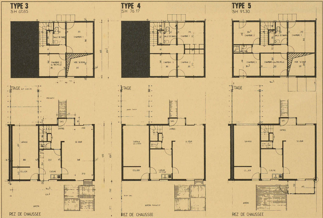
Plans-types du lauréat de « Villabois international ».
