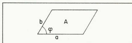
Fig. 7. — Surface du parallélogramme.
