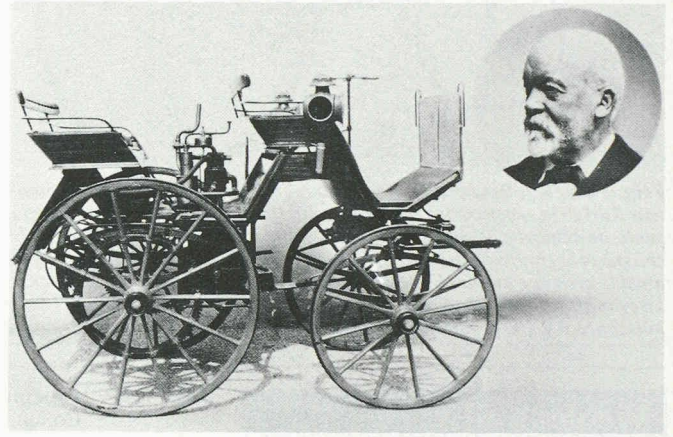
Calèche à moteur Daimler, construite en 1886. Une force invisible mouvait une calèche qui jusqu'alors était tirée par des chevaux ; on n'avait encore jamais vu cela. Elle était propulsée par le premier petit moteur léger et rapide à essence du monde de Gottlieb Daimler. Données techniques moteur Daimler : un cylindre vertical (refroidi par eau), alésage 70 mm, course 122 mm, cylindrée 469 cm 3 , puissance 1,5 CV à 700 tr/mn, vitesse maxi 16 km/h.
