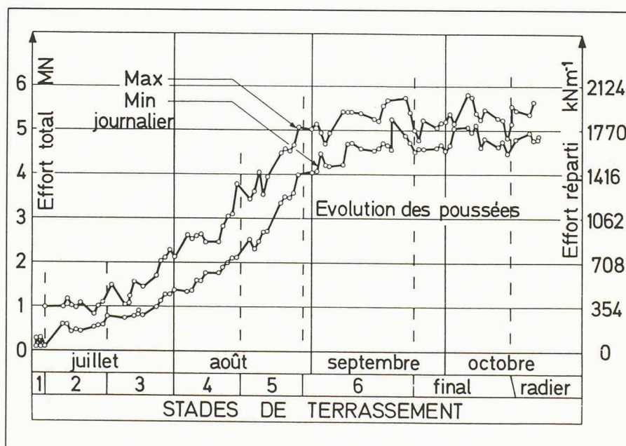
Fig. 5. — Confédération Centre. Fouille 4. Evolution des efforts totaux.
