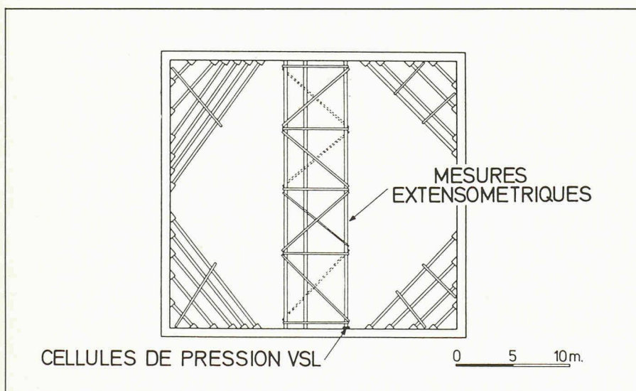
Fig. 3. — Confédération Centre. Fouille 4. Schéma d'étaisage et situation des points de mesure.
