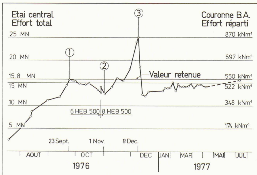
Fig. 10. — Grand Casino. Evolution des efforts sur l'étaï central.
