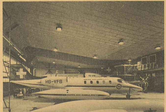
Garde aérienne suisse de sauvetage à Zurich : 1600 m 2 Schichtex-SW 75/III avec noyau en laine minérale, surface visible peinte au pistolet blanc-gris, posé dans des profils-doubles-T, suspendu avec supports spéciaux.
