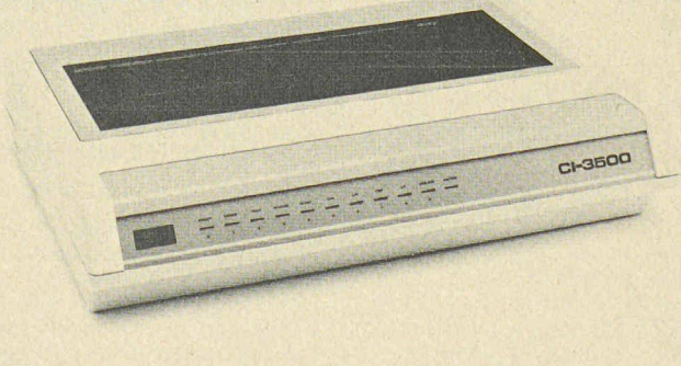
L'imprimante CI-3500 se présente sous une forme particulièrement compacte (hauteur 12 cm, largeur 57 cm, profondeur 42 cm). En cartouche: écriture en qualité courrier (vraie grandeur).
