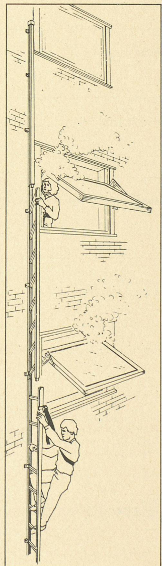
La nouvelle échelle de sauvetage incendie de la compagnie norvégienne Smijernprodukter a.s., Vikersund, ressemble à une barre contre une façade. Elle se déploie en une échelle stable lorsque le bouchon de blocage au sommet et à chaque étage est dégagé. L'échelle ne peut pas être ouverte du sol et ainsi assure également protection contre les cambrioleurs.
