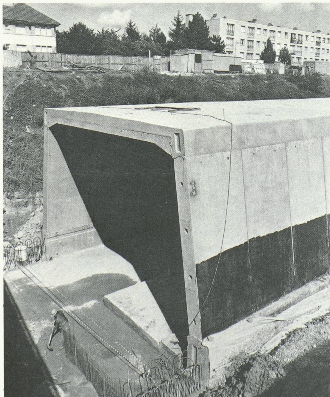
Élément de tranchée couverte, sur le même site que sur la photographie à droite en haut de page.
