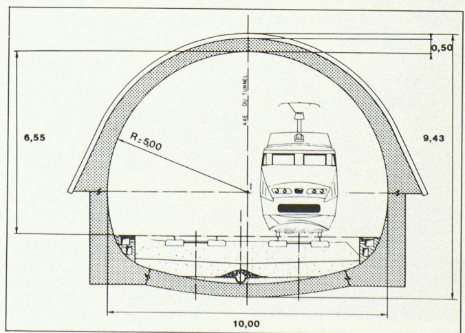
Section type des tunnels de Fontenay et de Sceaux (pour 200 km/h).
