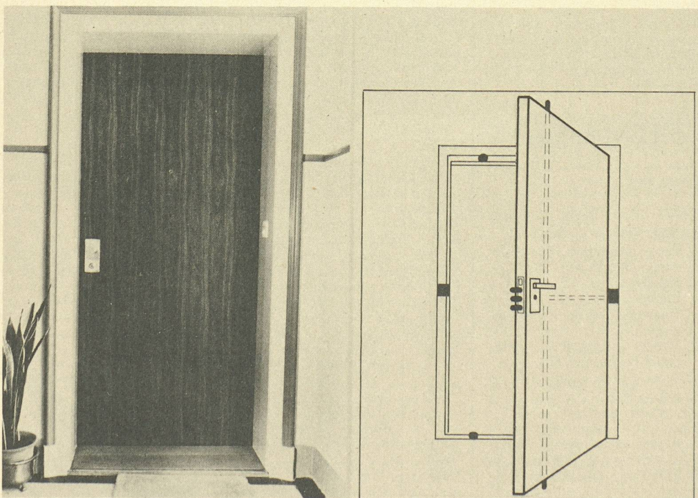
Le dispositif de sécurité Multilock se monte aisément sur toutes les portes, nouvelles ou existantes ; il est absolument invisible tant de l'extérieur que de l'intérieur (photo de gauche). Le dessin à droite montre comment le système fonctionne : la porte, verrouillée des quatre côtés au moyen de barres de blocage, offre une protection maximale contre les effractions.
