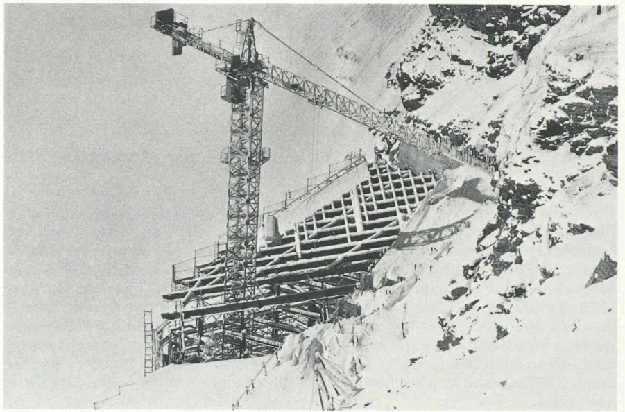
Fig. 11. — L'utilisation de grues a préalablement nécessité la création de solides points de fixation (socle de béton: 140\text{ m}^3 ).
