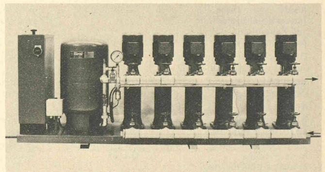
Surpresseur automatique Biral DWA-P commandé par microprocesseur pour l'amortissement des coups de béliet dans les réseaux fortement sollicités.
