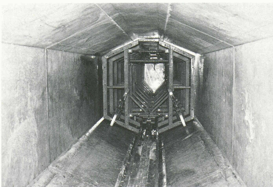
Fig. 5. — Le coffrage à l'extrémité d'une section terminée.
