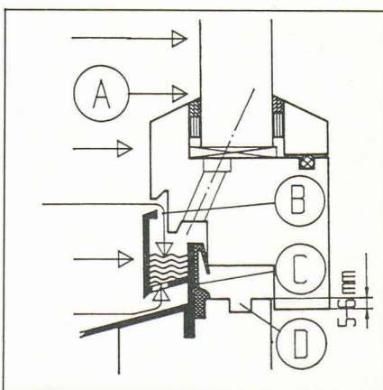
Fig. 3. — Evacuation de l'eau de pluie. A: Pression du vent. B: Joint de décompression. C: Etanchéité centrale. D: Rainure pour les ferrants.
