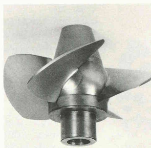
Roue modèle réduit d'une turbine Kaplan.
