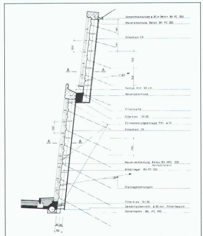
Coupe type de la paroi ancrée.
