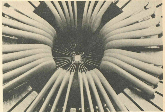
Test aux frontières de la technique au centre de recherche IBM de Yorktown Heights, dans l'Etat de New York. Semblables aux pétales d'une marguerite électronique, les tiges des électrodes de l'équipement de test rayonnent autour d'une microplaquette de silicium sur laquelle sont implantés les plus petits transistors du monde. Présenant des composants inférieurs au dixième de micromètre, soit mille fois plus minces qu'un cheveu, ces transistors pourraient servir à la construction d'ordinateurs atteignant plusieurs fois la puissance maximale envisagée jusqu'à présent.
