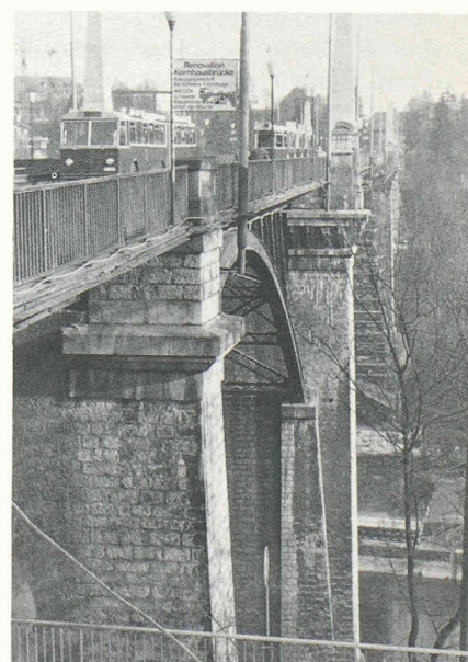
Fig. 6. — Piles salies, garde-fou corrodé.
