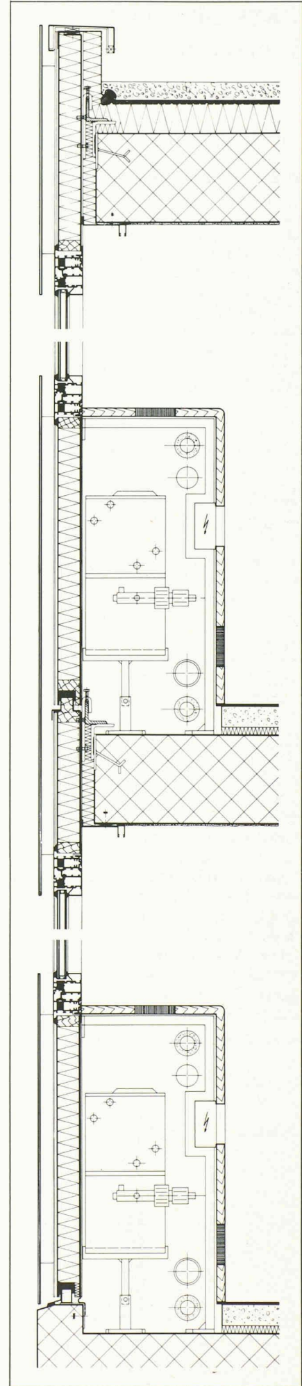
Coupe verticale.
