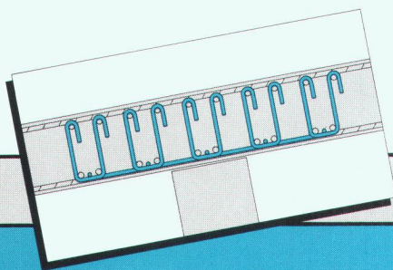
Disposition de l'armature dans un panier de poinçonnement Dura.
