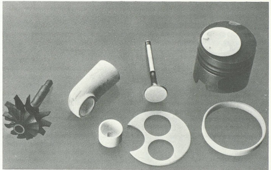
Fig. 2. - Eléments de moteur en céramique.
