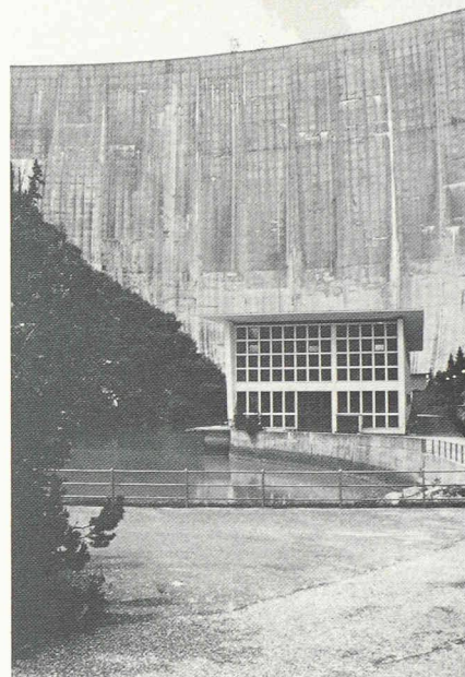
Vue aval du barrage de Zervreila. Au premier plan, le bâtiment de l'usine du lac. La prise de la conduite d'amenée aux turbines est située 23,5 m au-dessus du niveau minimal de la retenue. Devant l'usine, on a construit un bassin de compensation qui permet de faire passer l'eau de la vallée de Vals à celle de Safien, dans une galerie en charge. Ce bassin sert également de bassin de pompage pour refouler l'eau supplémentaire du torrent Peiler dans le lac artificiel durant l'été. Avec deux turbines Francis d'un débit global de 20 m 3 /s, l'usine du lac de Zervreila produit environ 15 GWh d'énergie d'hiver de haute valeur.
