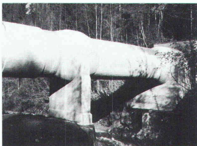
Siphon Rempen, Centrale Hydroélectrique de Wägital AG
