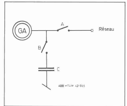
Fig. 5. - Compensation par condensateur pour une machine asynchrone.
