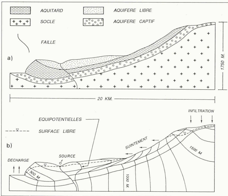
Fig. 1. - Ecoulement variablement saturé dans un système multicouche complexe. a) Structure du domaine d'écoulement b) Equipotentiels et surface de la nappe libre
