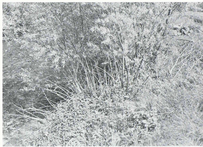
Fig. 7. – Technique du peigne. (a) Des arbres et buissons branchus sont placés dans la niche d'érosion (1984). (b) Les éléments en suspension dans l'eau sont retenus par effet de filtre dans les branches lors de la crue (1985). (c) La berge se reconstitue par accumulation des sédiments et la végétation du «peigne» se développe en contribuant à la fixation de la berge (1991).
